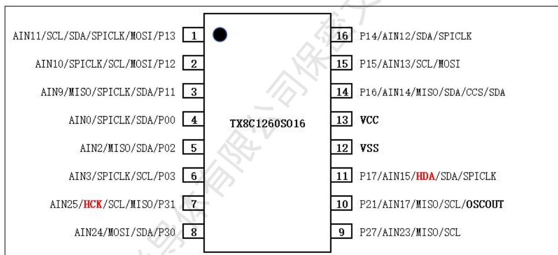
图 8 - TX8C1260S016 (SOP16) 封装图
